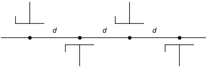
Fig. 1.9. Glide-plane symmetry
